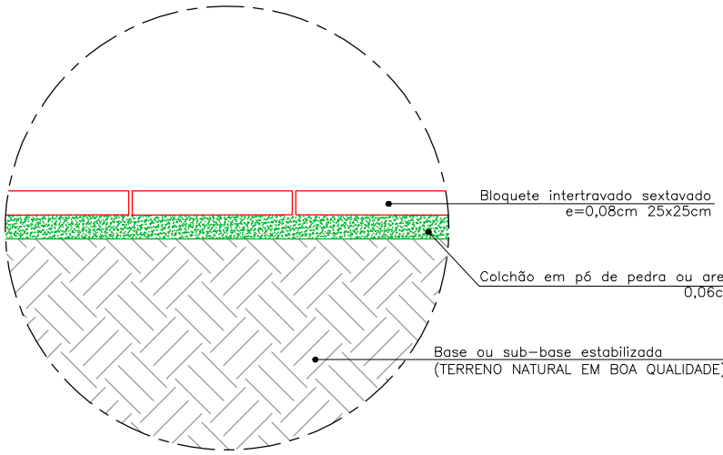
Det. 02 - Calçamento Sem escala
